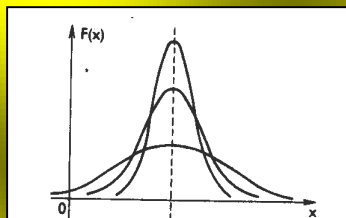
Charakteristické priebehy Gausovej krivky . Na ose x sú hodnoty meranej (hodnotenej) veličiny, na ose y je ich frekvencia (početnosť). Je iba vecou konvencie, aké hodnoty (na ose x ) sa zvolia za hranice „normy“, resp. „priemeru“ (napr. v našom prípade „strednej vrstvy“).
